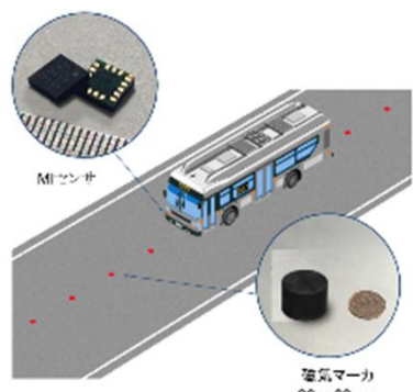
▲磁気マーカ設置イメージ
